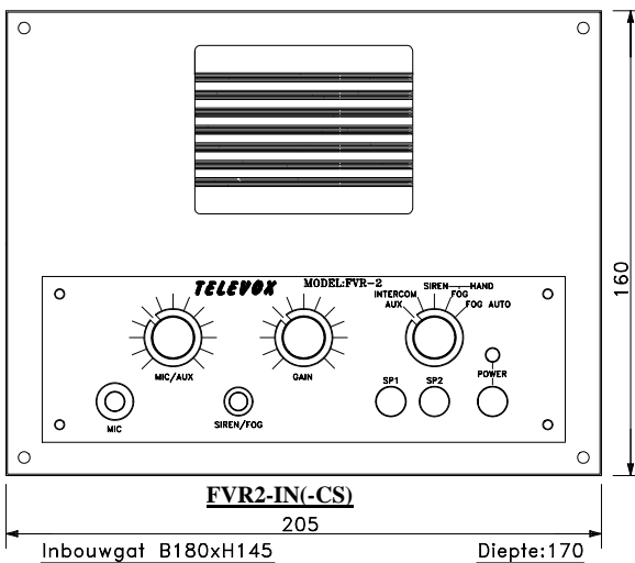
Inbouwgat B180xH145
